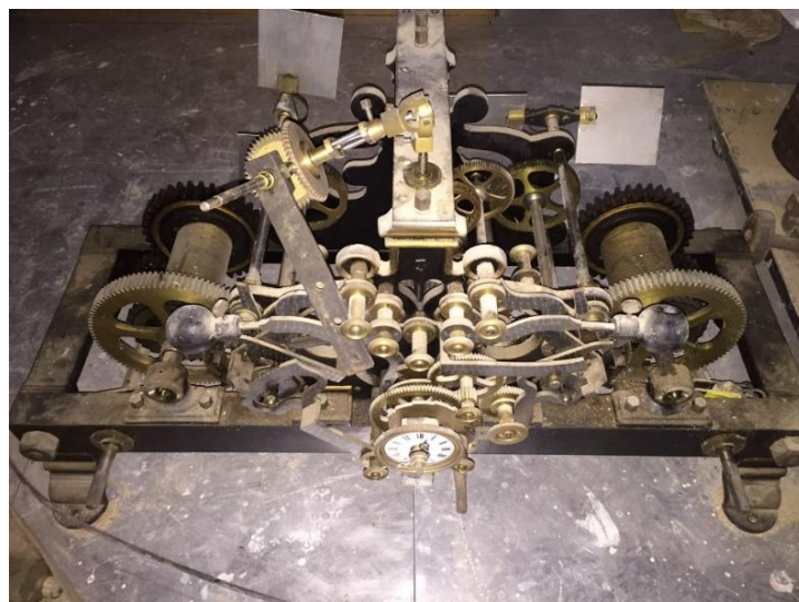
Le mécanisme Francis Paget avant restauration.
