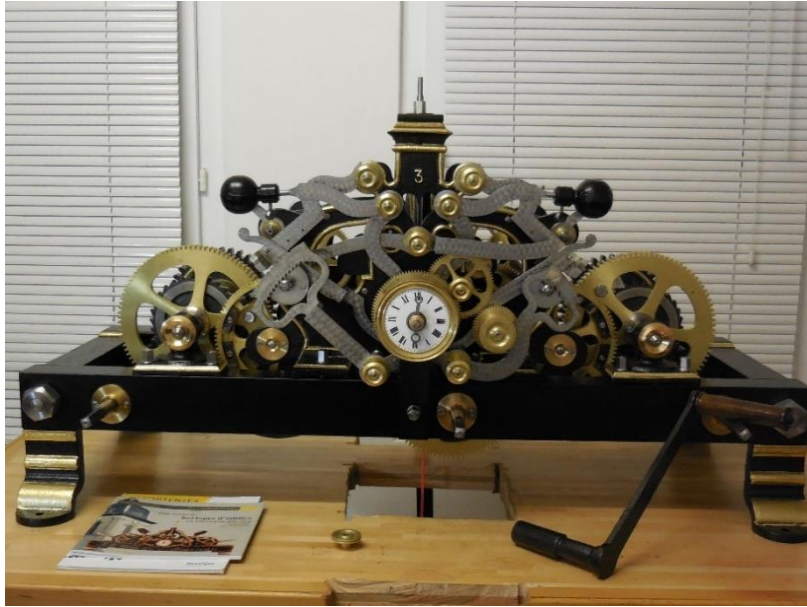
Le mécanisme après restauration.
